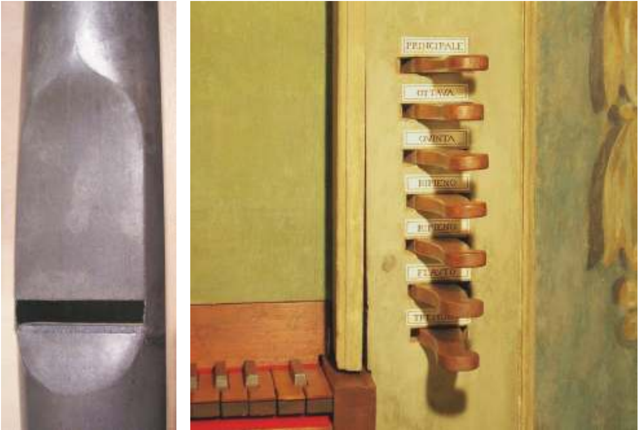
Particolare della canna centrale di facciata e dei comandi di registrazione.
